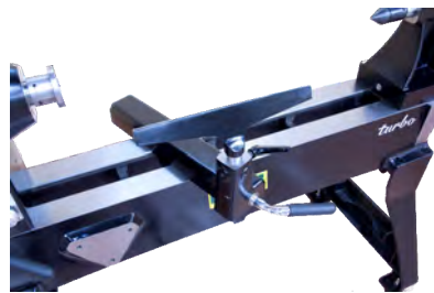
Handauflage mit Schnellverschluss
