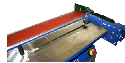
Schleifbandkipfung 90 Grad
