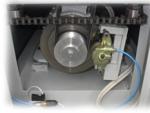
schwere Kraftübertragungselemente
